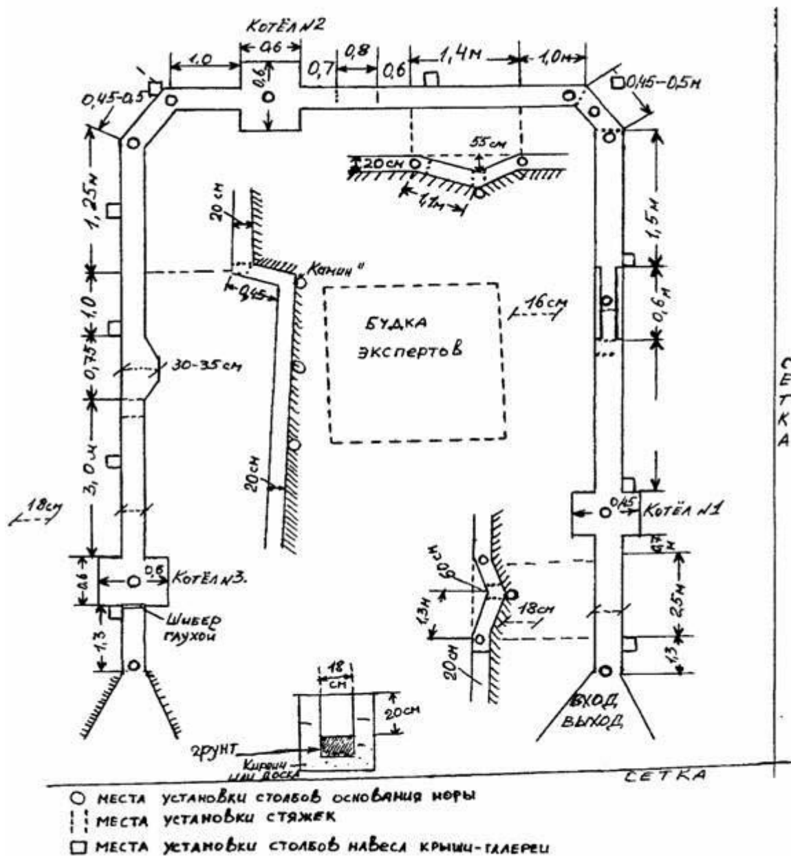
Схема П-образной норы для испытаний собак по лисице и барсуку
